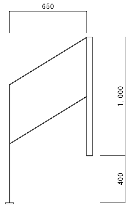
アイアン手摺立面
