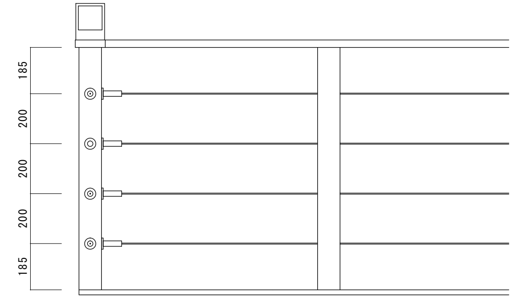
オープンデッキ フェンス・ベンチ詳細 1:15
