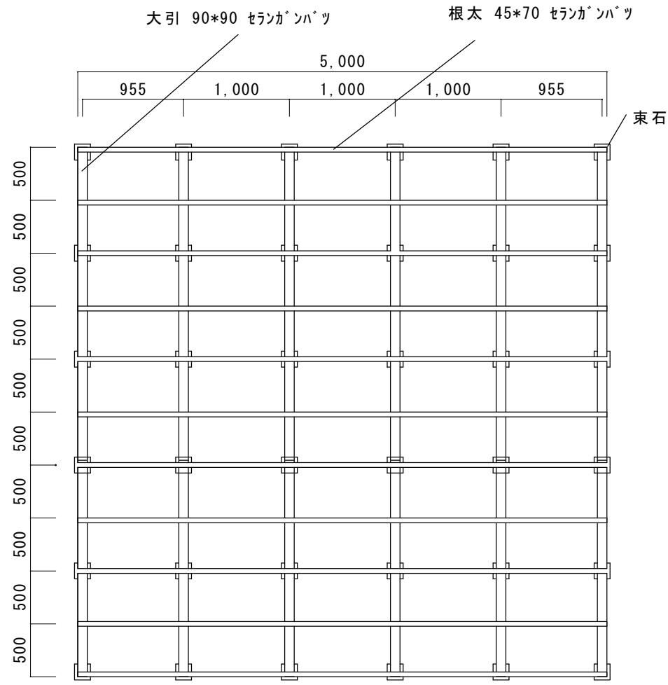
オープンデッキ 1:50
